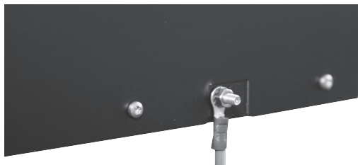
Korrekt angeschlossener Schutzleiter
