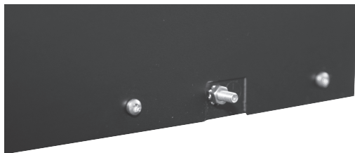
Schutzleiteranschlussbolzen
